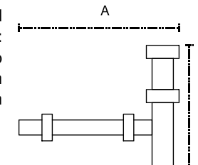
Sifón Recto Mod. 90.0093
