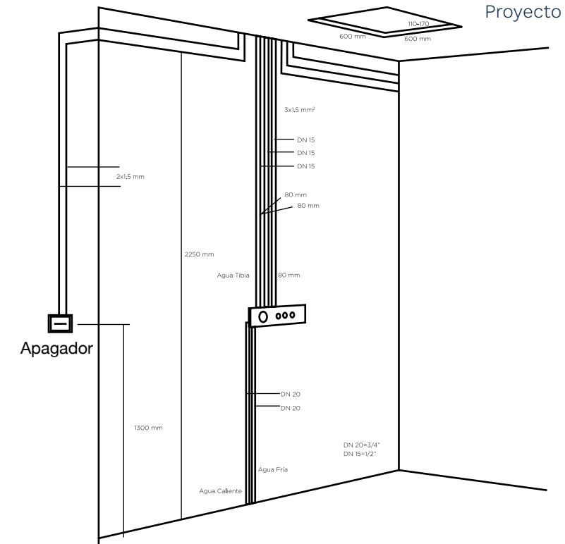
Brazo a Pared regadera de alta presión Mod. 5450401CR
